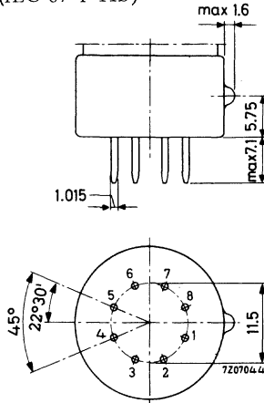
RIMLOCK BASE (IEC 67-1-11b)
